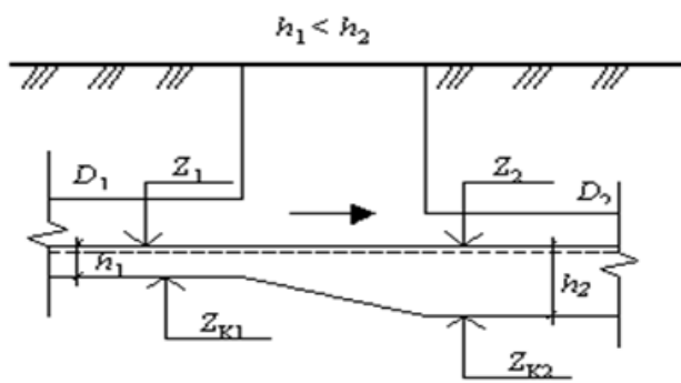
Рисунок А.2. Соединение трубопровод по уровню воды
