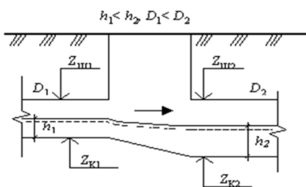
Рисунок А.1. Соединение трубопровод по шельгам
