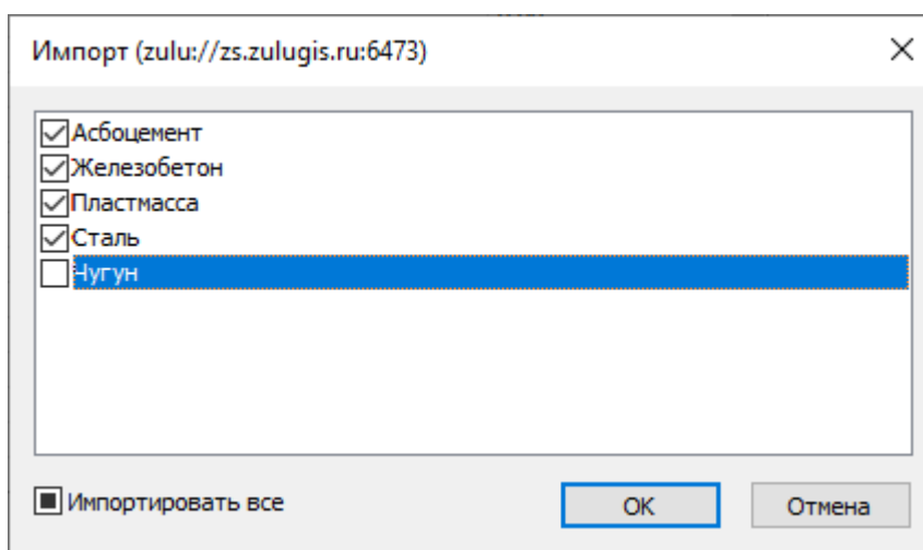
Рисунок 21.14. Импорт сортаментов
