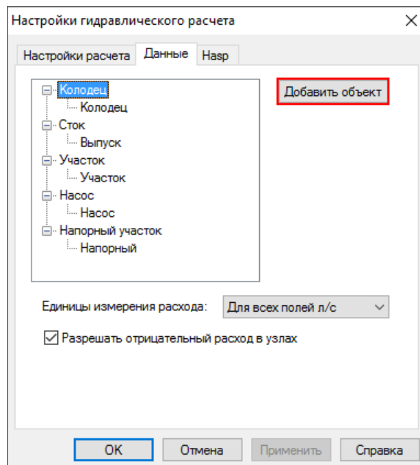
Рисунок 8.4. Добавление объекта
