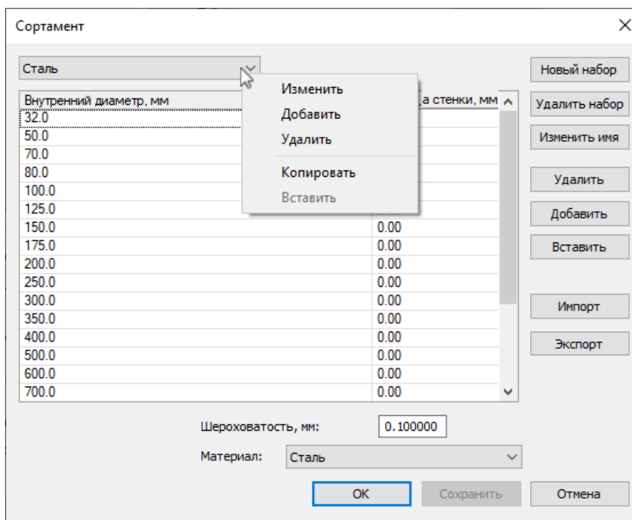
Рисунок 21.8. Копирование сортамента
