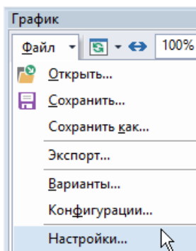
Рисунок 15.13. Настройки графика
