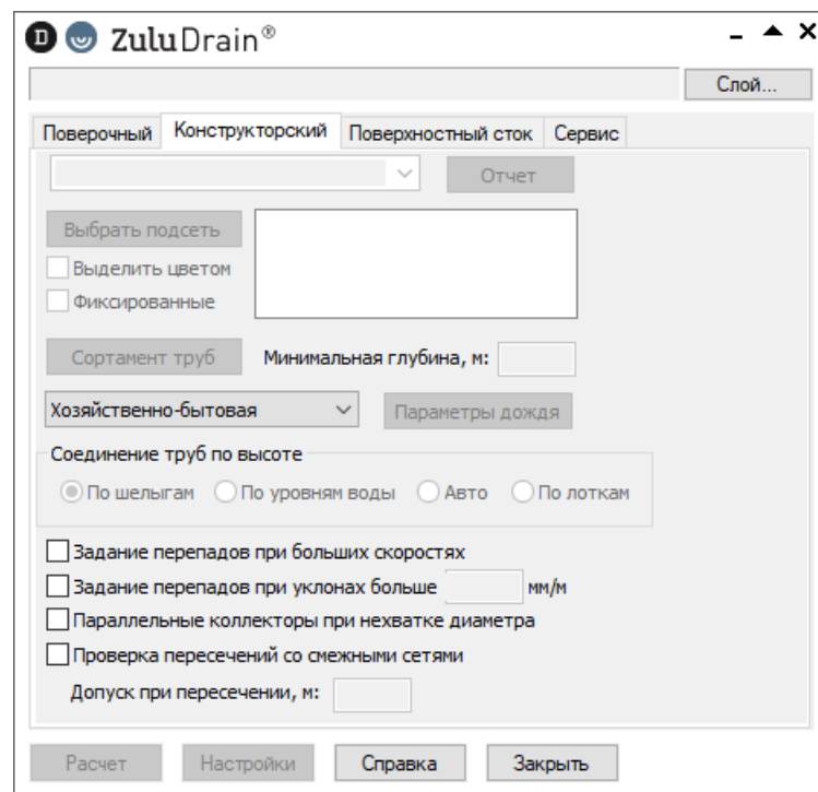
Рисунок 11.3. Панель расчетов
