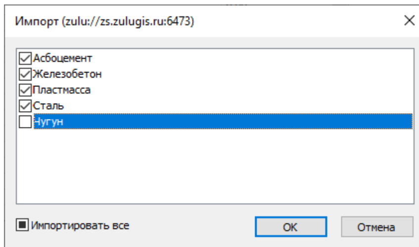
Рисунок 21.12. Импорт сортаментов
