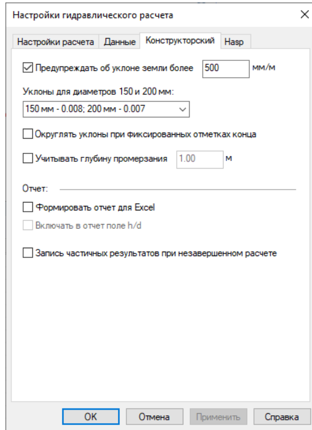
Рисунок 11.6. Вкладка Конструкторский
