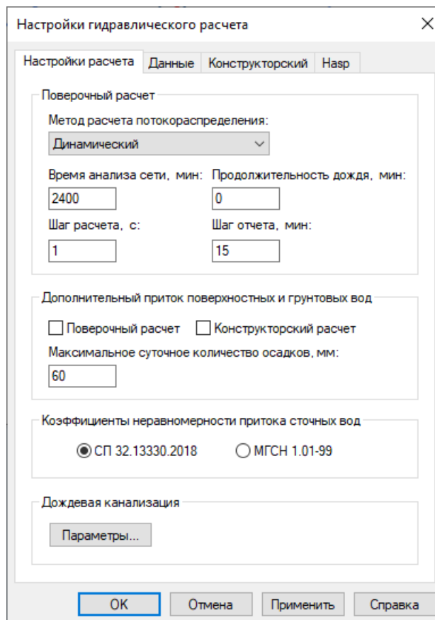
Рисунок 12.10. Настройки расчета
