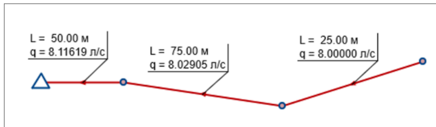
Рисунок Е.2. Пример схемы
