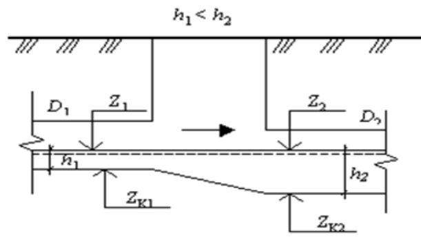
Рисунок А.3. Соединение трубопровод по лоткам
