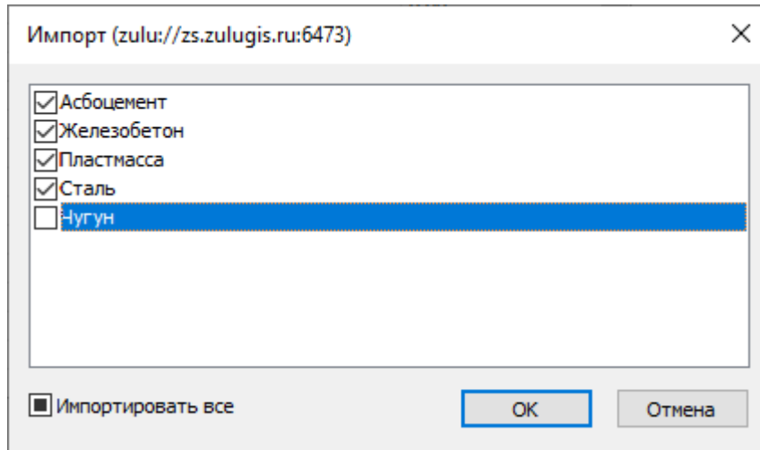
Рисунок 21.19. Импорт сортаментов
