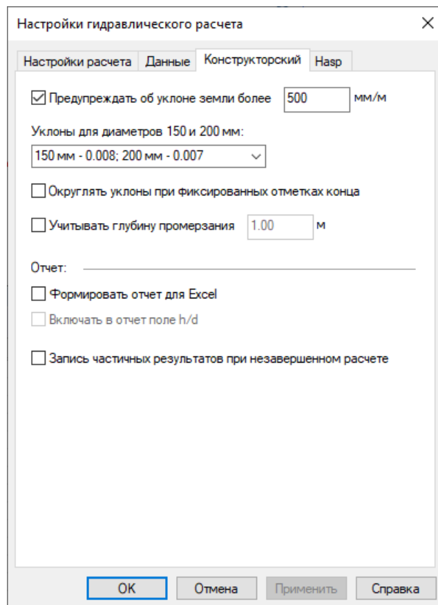
Рисунок 12.12. Вкладка Конструкторский
