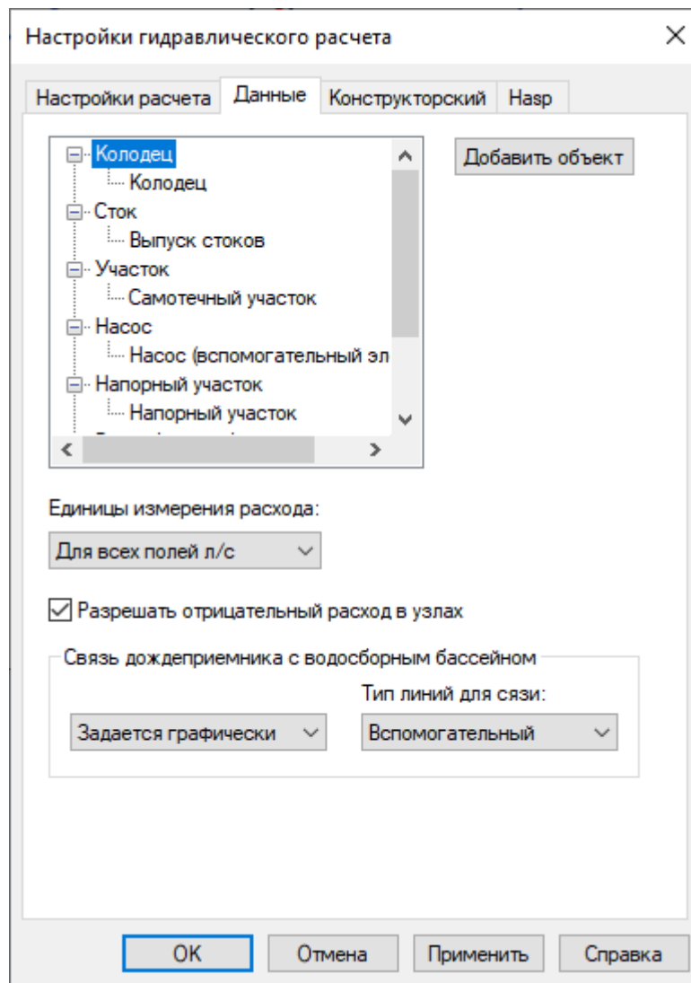
Рисунок 12.11. Вкладка Данные
