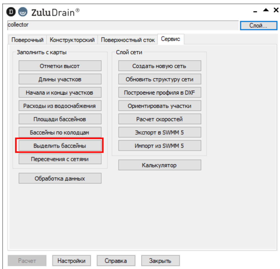
Рисунок 19.19. Вкладка Сервис
