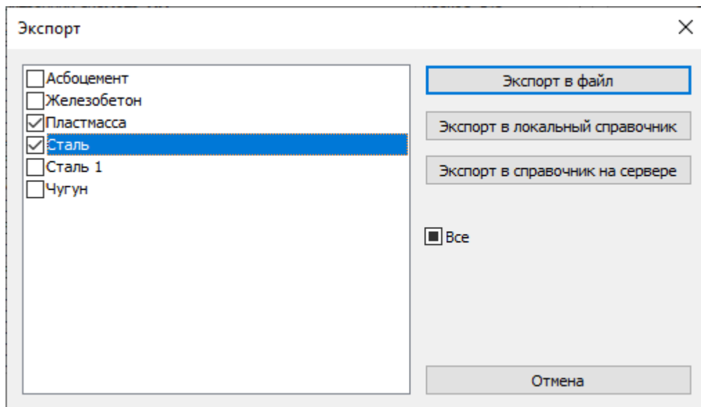
Рисунок 21.20. Экспорт сортаментов
