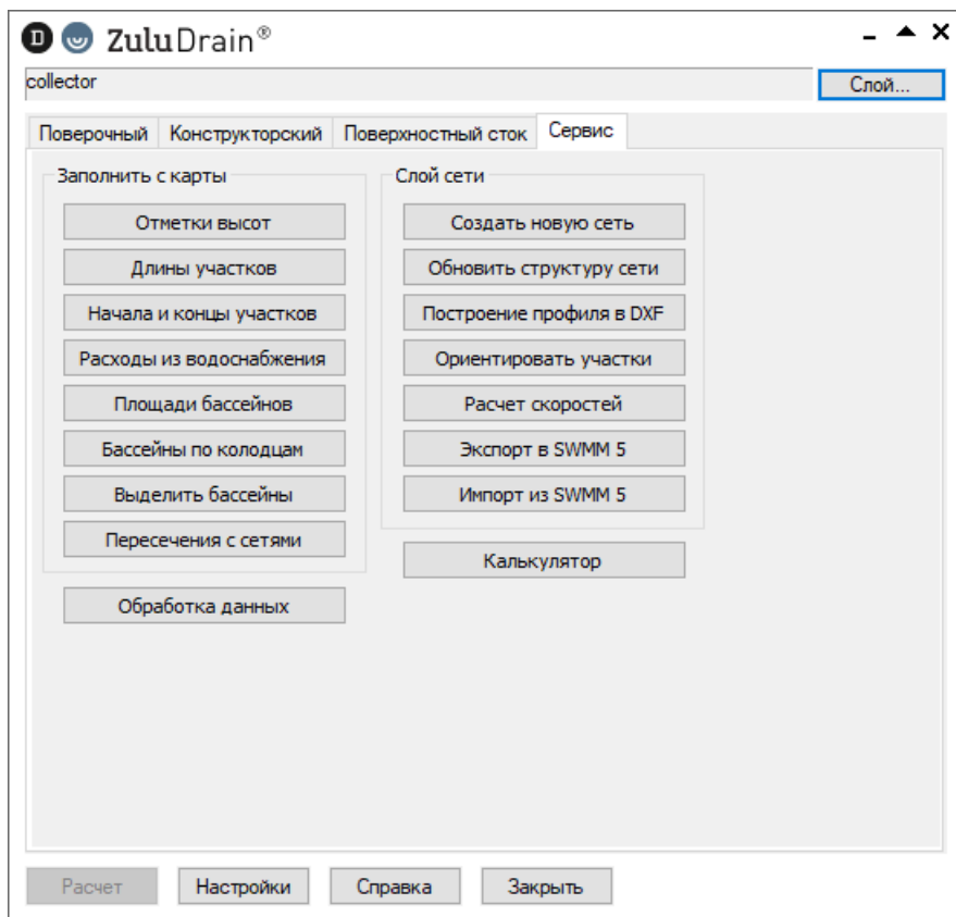
Рисунок 23.4. Вкладка Сервис
