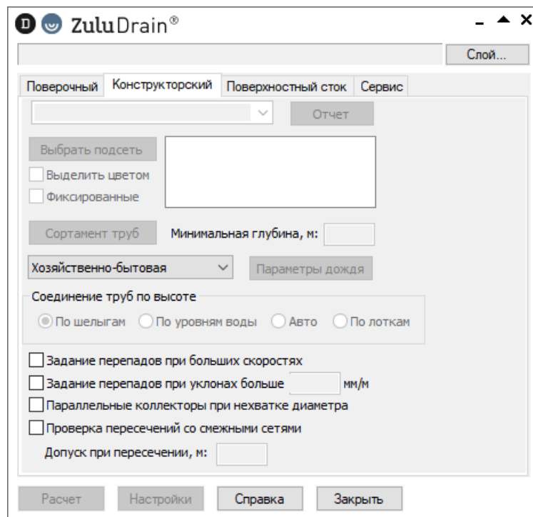
Рисунок 12.9. Панель расчетов
