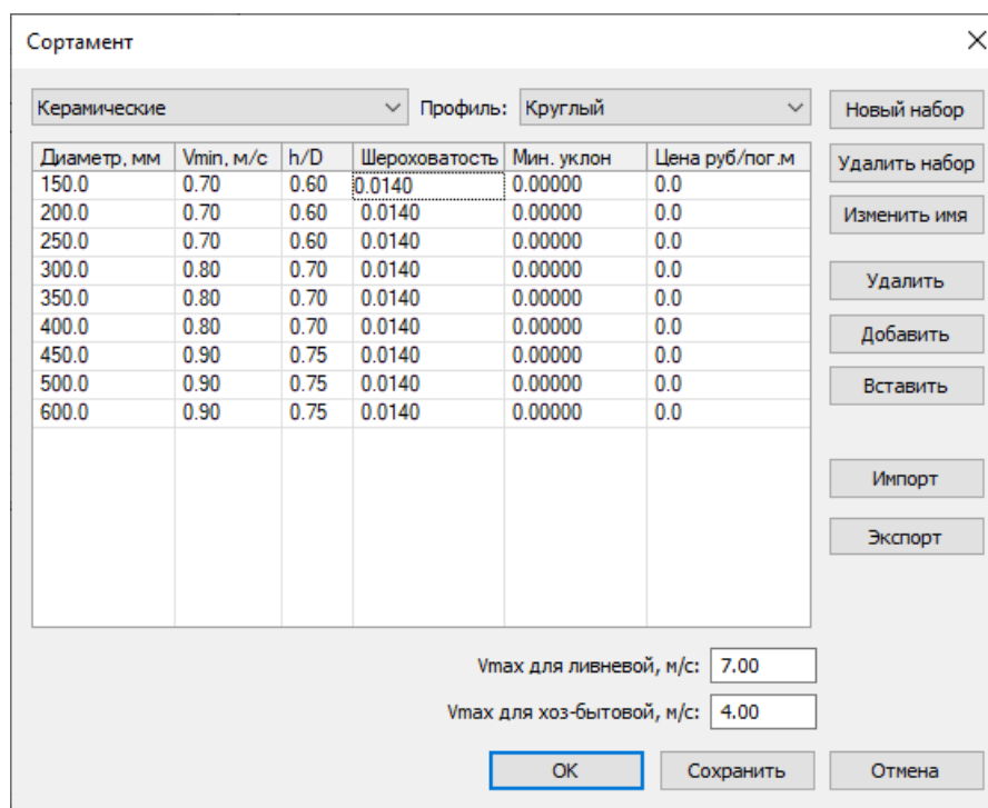
Рисунок 21.3. Окно «Сортамент»
