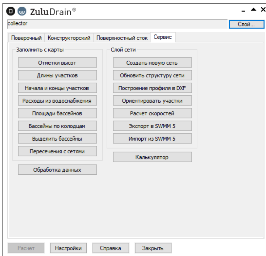
Рисунок 9.1. Вкладка Сервис
