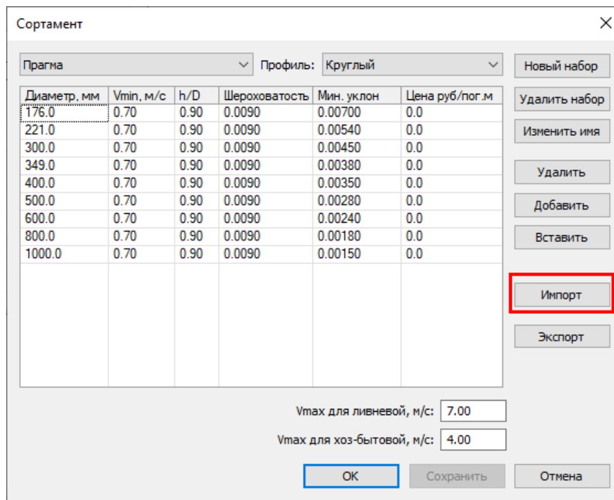
Рисунок 21.9. Импорт сортамента
